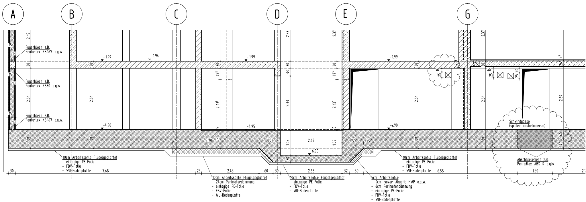
Schnitt A-A
