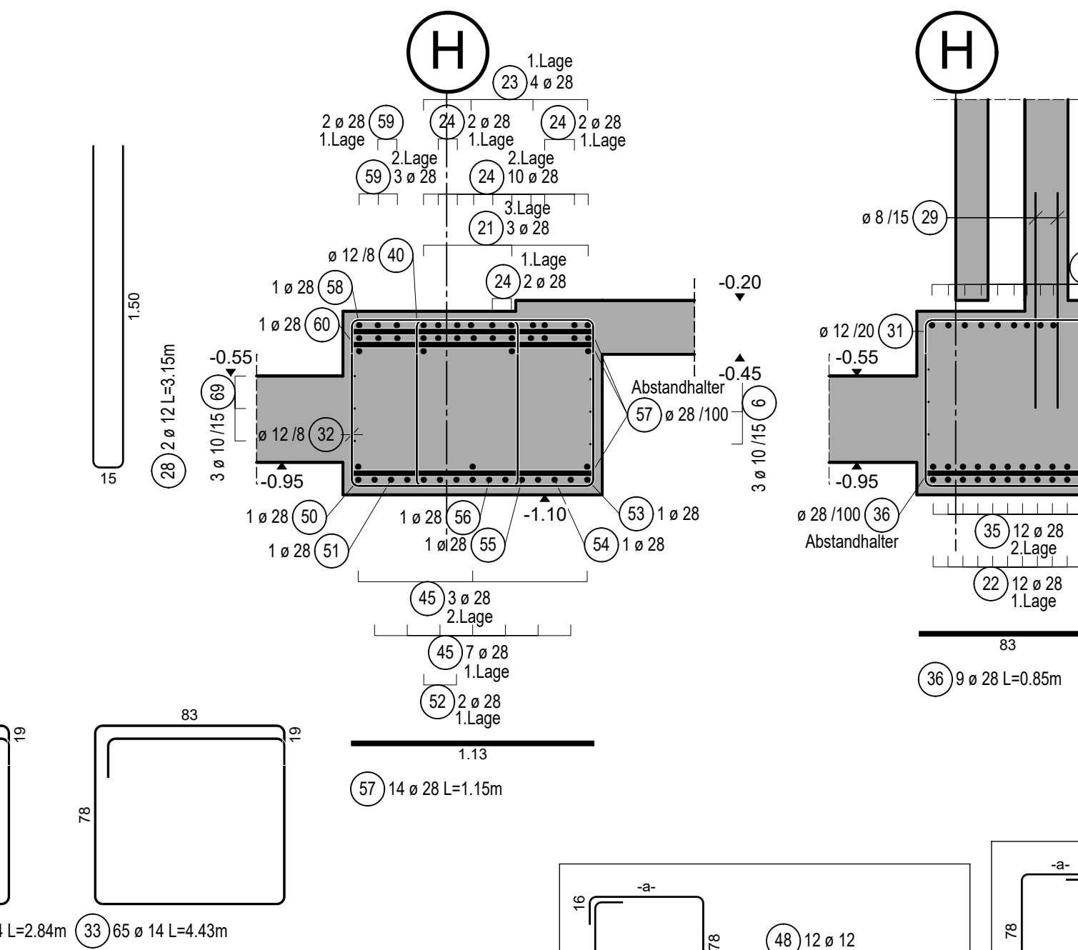
Schnitt 6-6, M1:25
