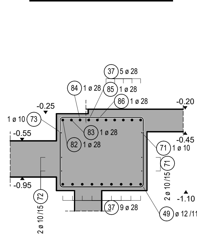
Schnitt 8-8, M1:25
