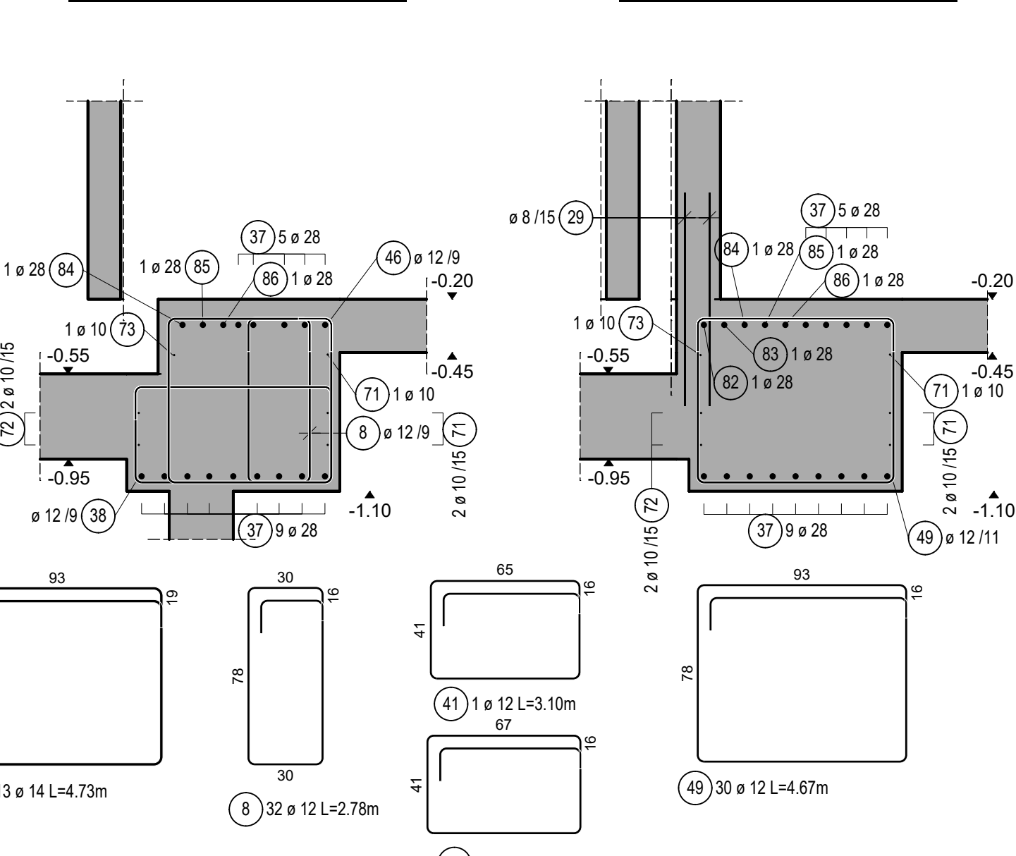
Schnitt 4-4, M1:25
