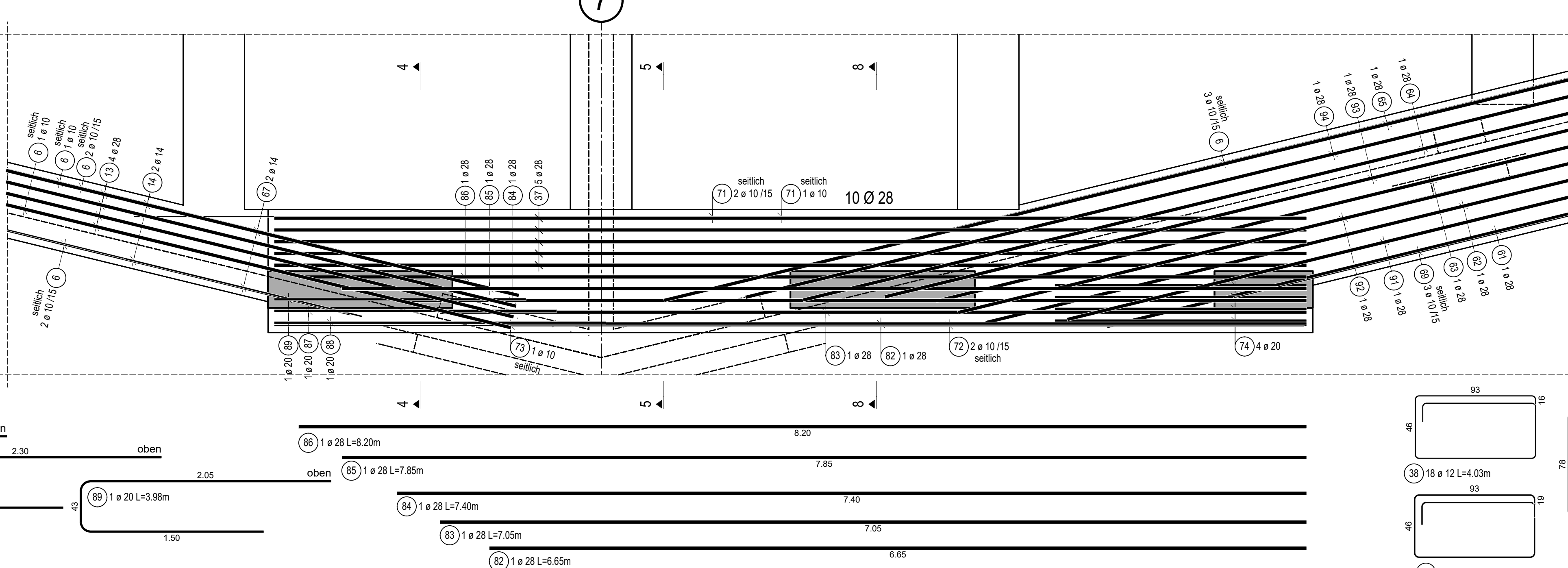
obere Lage und Randbewehrung
