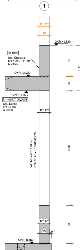
Schnitt SP-EG-01-07 M.: 1 : 25
