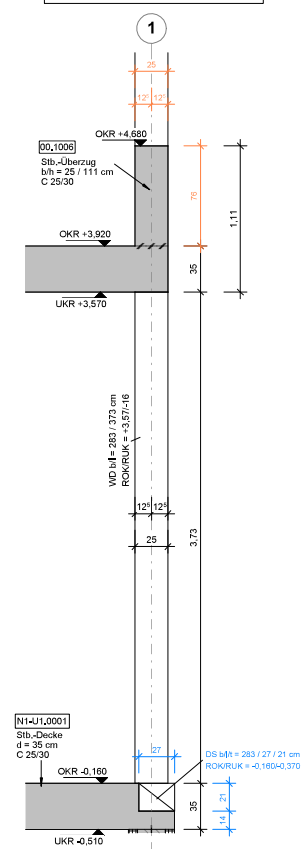
Schnitt SP-EG-01-08 M.: 1 : 25
