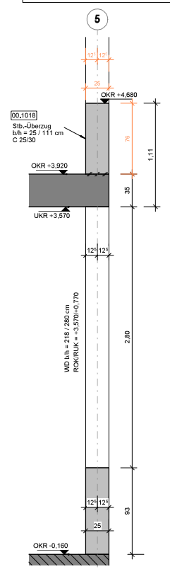
Schnitt SP-EG-01-09 M.: 1 : 25
