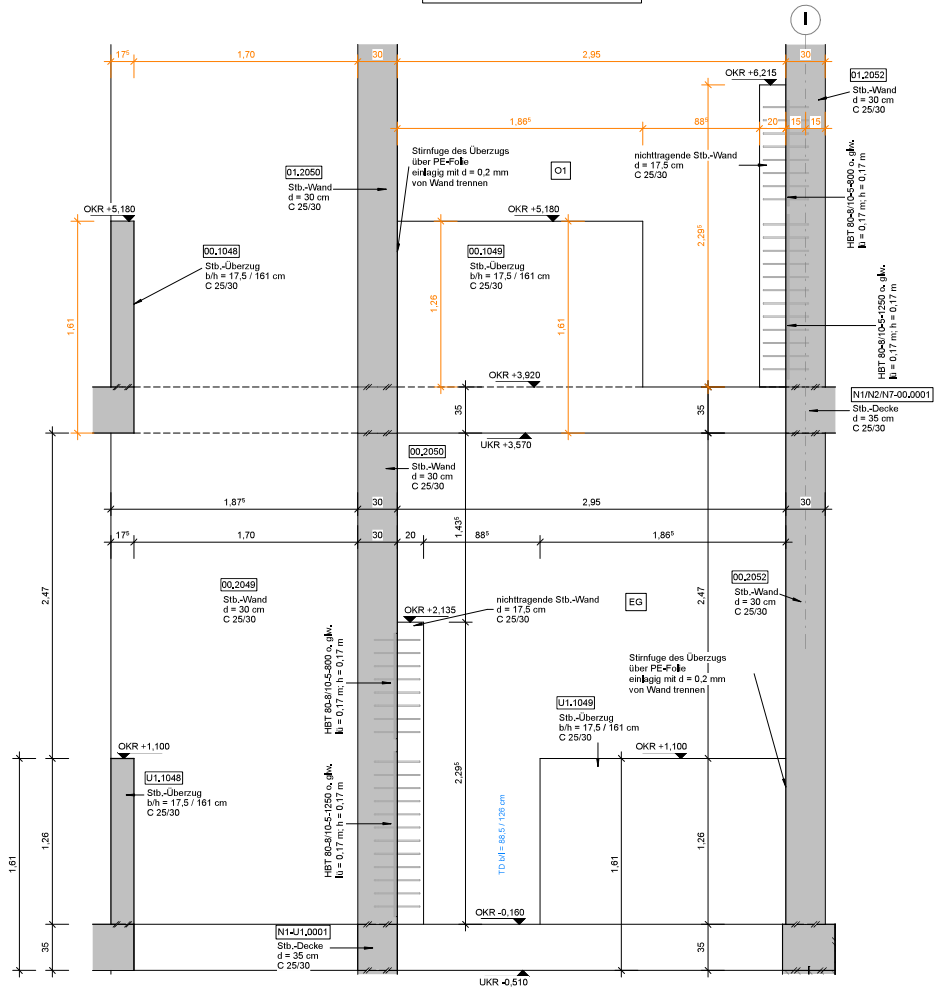
Schnitt SP-EG-01-06 M.: 1 : 25
